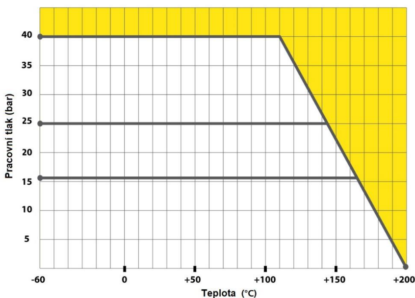
Diagram závislosti maximálního přípustného tlaku na teplotě
